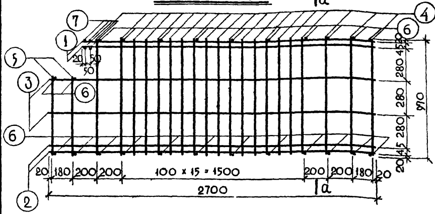
КАРКАС К-2 1б
