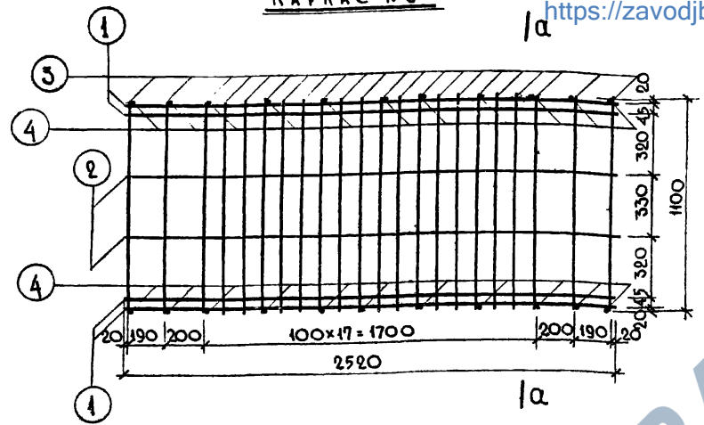
КАРКАС К-8
