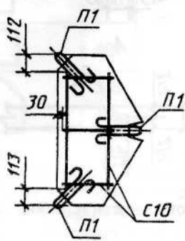
Армирование тротуарной плиты 11Д
