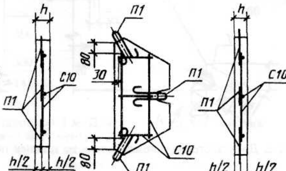
Армирование тротуарной плиты 14Д
